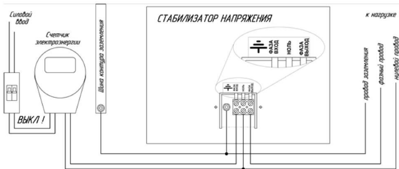
Рисунок 2. Рекомендуемая схема подключения стабилизатора к сети.
