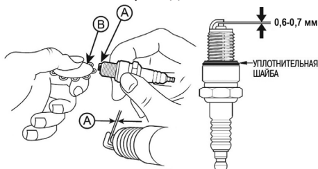
Рис. 20 Проверка зазора между электродами А – зазор В – щуп
