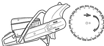
Рис. 5 Проверка направления вращения диска
