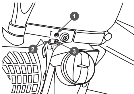
Рис. 19 Винты регулировки карбюратора 1 - винт «Т», 2 - винт «L», 3 - винт «H»
