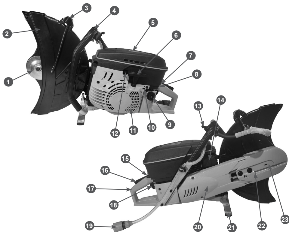
Рис. 3 Основные узлы и органы управления
