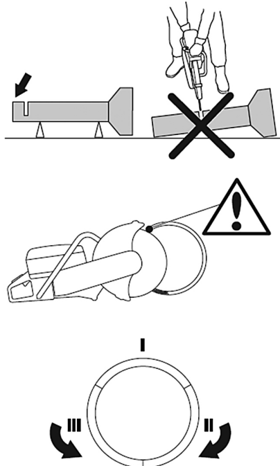
Рис. 15 Резка труб
