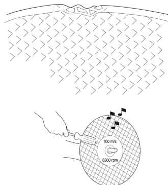
Рис. 9 Проверка абразивного диска
